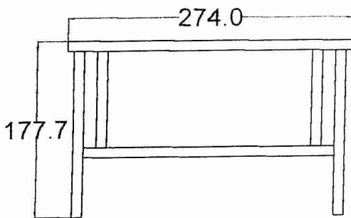
POGLED 1 - ploča za crtanje i pisanje
